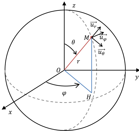
Document 2 – coordonnées sphériques et déplacement élémentaire d\overrightarrow{OM}
