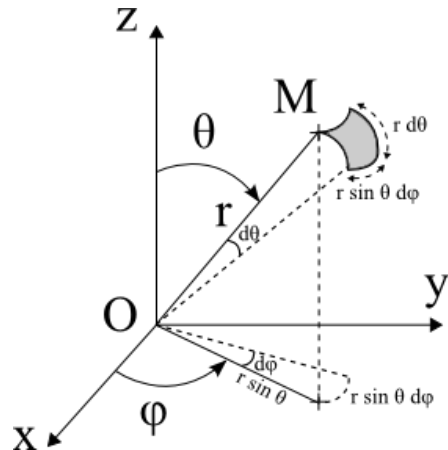
Document 2 – coordonnées sphériques et déplacement élémentaire d\overrightarrow{OM}
